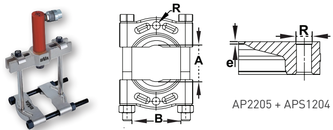
AP2205
